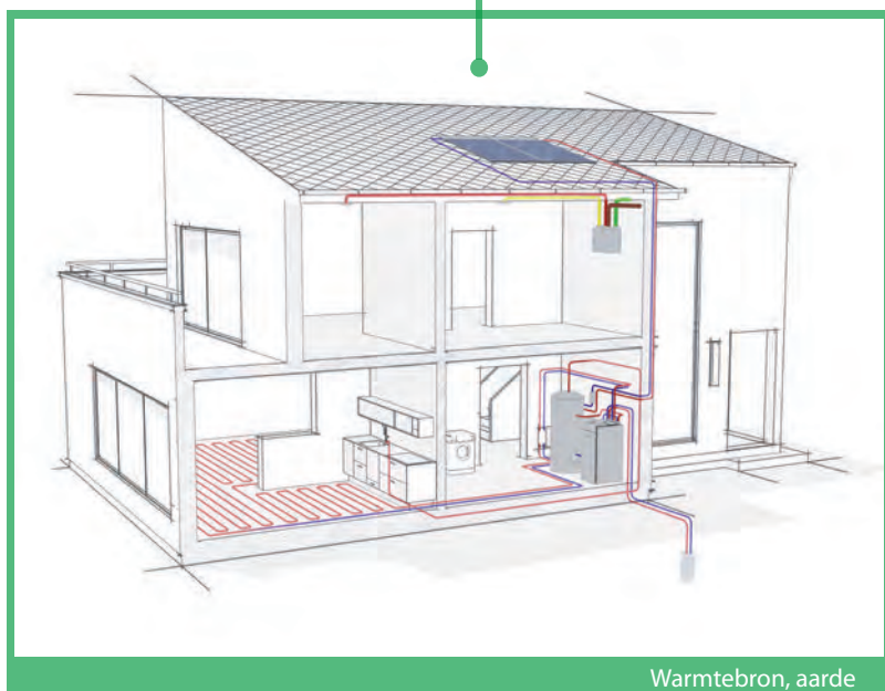
Warmtebron, aarde
